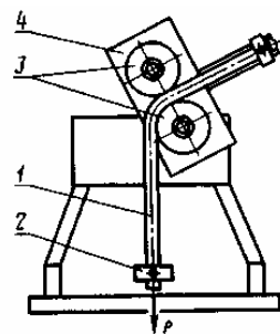
1 — испытуемый образец; 2 — груз; 3 — сменные ролики; 4 — пластина
