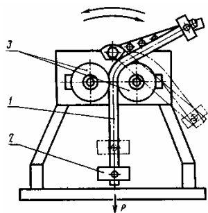
1 — испытуемый образец; 2 — груз; 3 — сменные ролики
